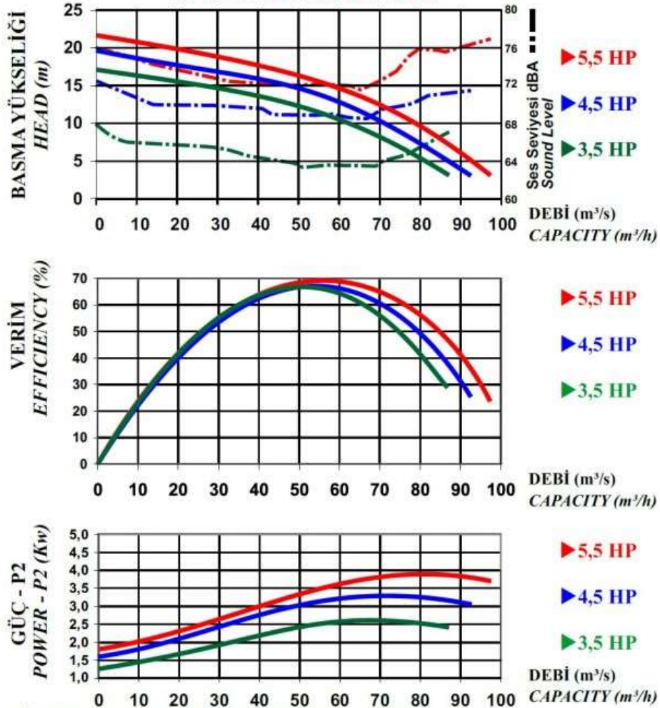
3,5 - 4,5 - 5,5 HP PERFORMANS EĞRİLERİ 3,5 - 4,5 - 5,5 HP PERFORMANCE RANGE
